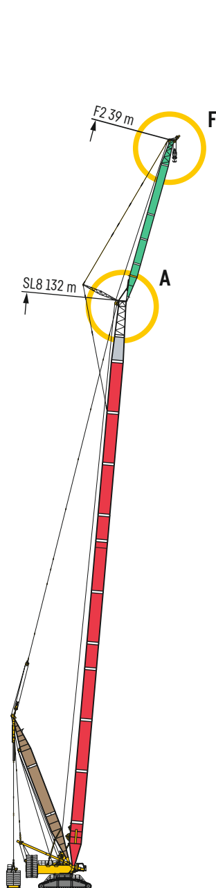
SL8DF2B SL8 102 m - 132 m F2 12 m - 39 m D 36 m
